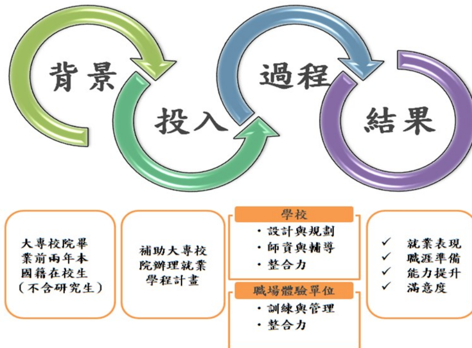
圖 2：評鑑架構圖
